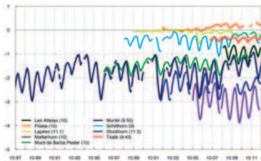
Graphique 5: Température du pergélisol Températures mesurées à environ 10 m de profondeur dans différents puits forés du réseau PERMOS. Graphique: Permos
