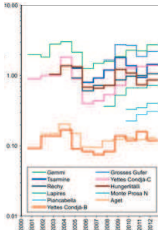
Graphique 6: Vitesses des glaciers rocheux: Vitesses de glissement horizontal de onze glaciers rocheux des Alpes suisses entre 2000 et 2012. Pour chaque glacier, la vitesse est déterminée par plusieurs points (de 5 à 30), relevés au moins une fois par année. La valeur indiquée est la valeur moyenne de tous les points de mesures. Graphique: Permos
